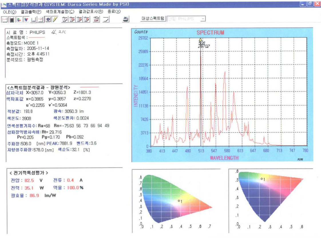
Philips D2S 86,9 Lm/W 3050 Lumen
