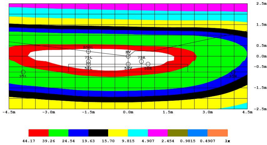
Horisontell ljusbild - Lux (lx)
