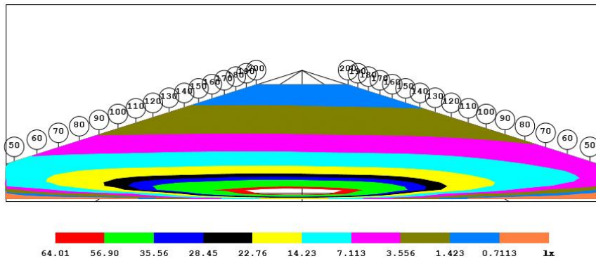
Horisontell ljusbild - Lux (lx)
