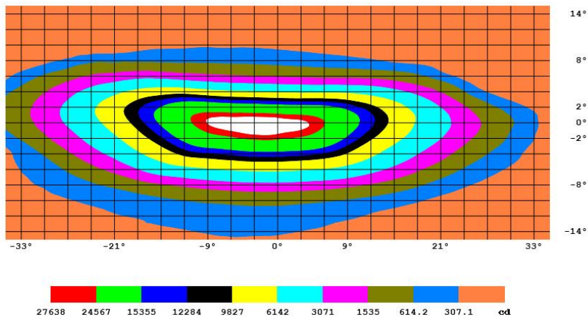
Vertikal ljusbild - Candela (cd)
